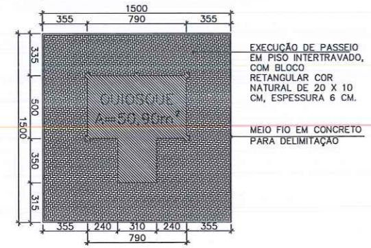
IMPLANTAÇÃO QUIOSQUE ESC.: 1/200
