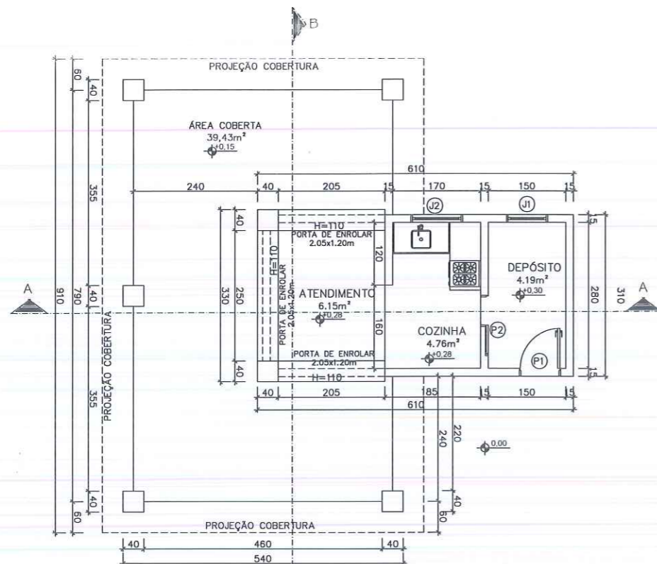
PLANTA BAIXA QUIOSQUE ESC.: 1/50 ÁREA=50,90m²
