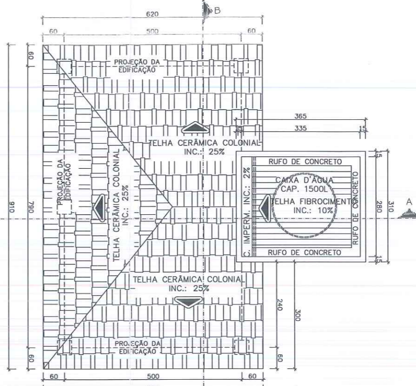
PLANTA DE COBERTURA ESC.: 1/50
